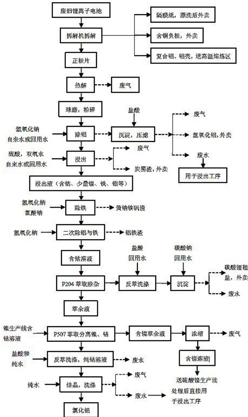
氯化钴生产线工艺流程图
