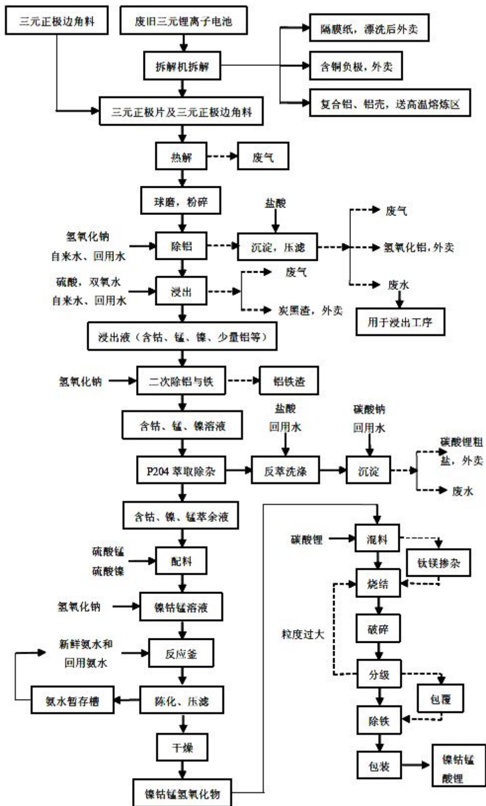
镍钴锰酸锂生产线工艺流程图
