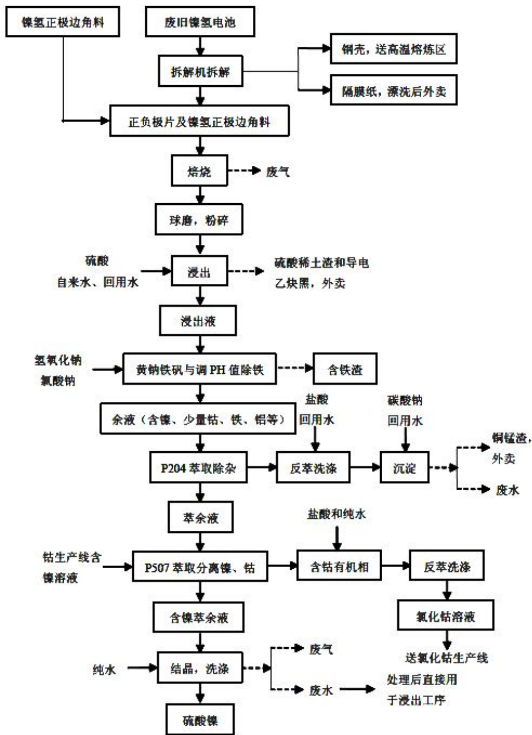
硫酸镍生产线工艺流程图
